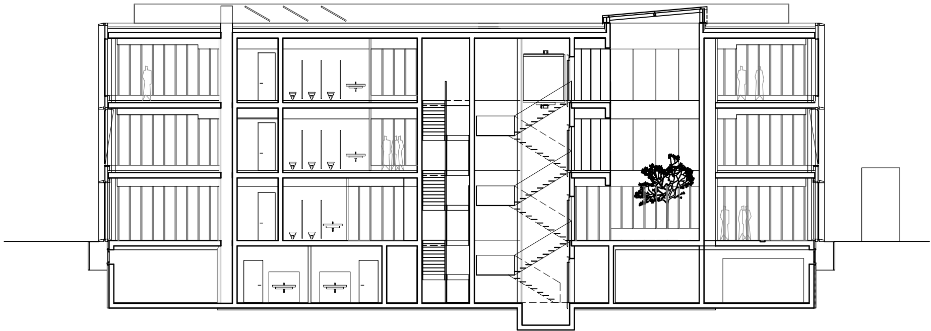
coupe longitudinale
