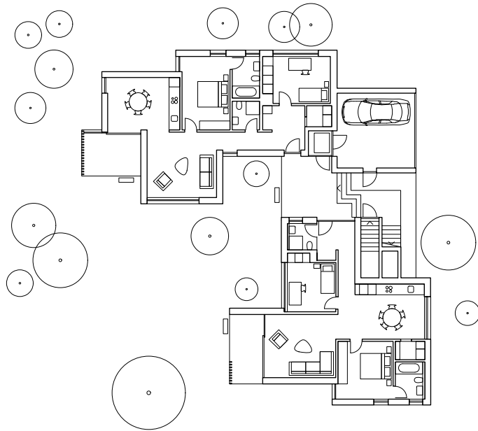
Grundriss Erdgeschoss
